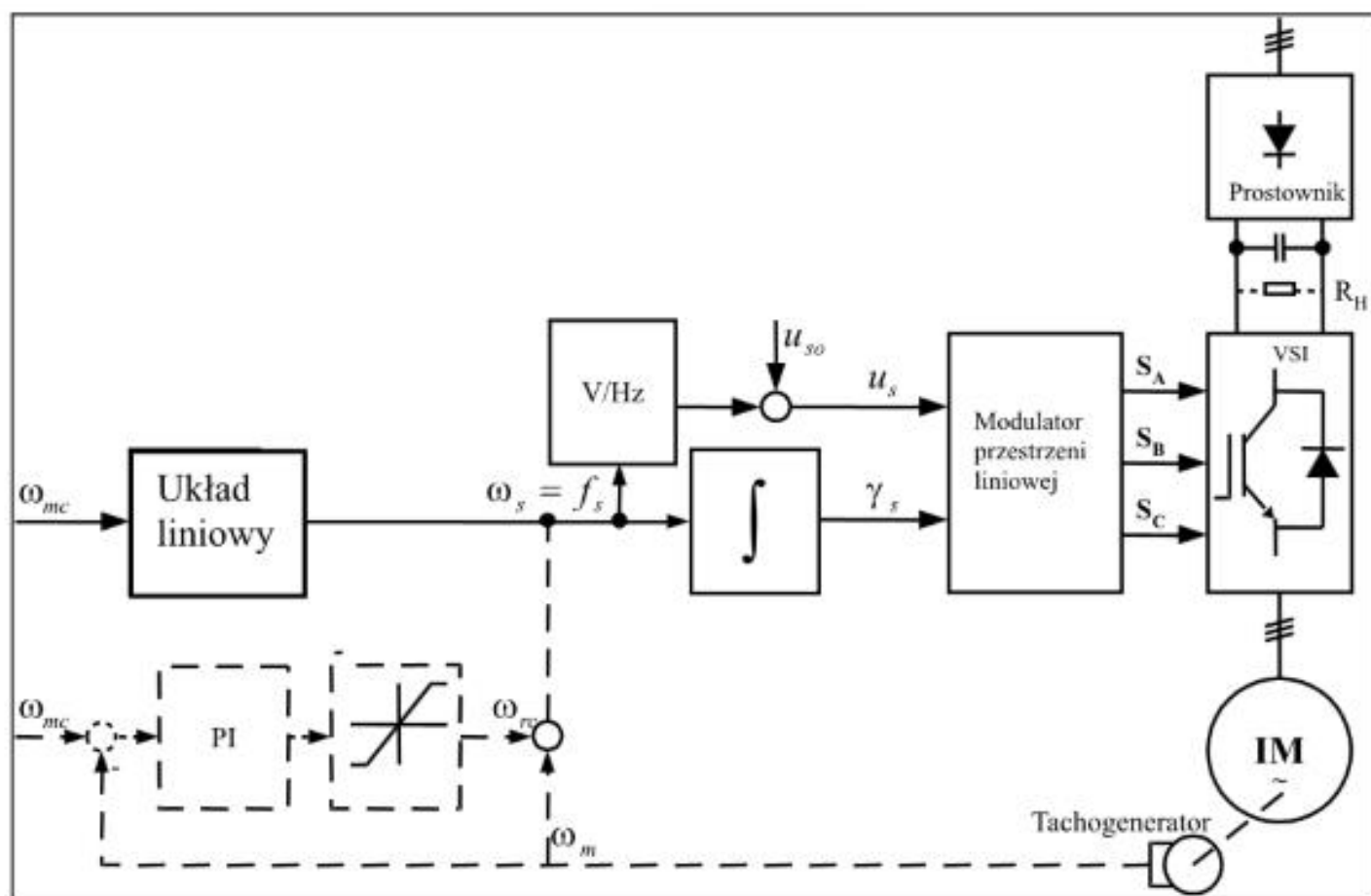
Rys. 3.3. Sterowanie skalarne typu u/f = \text{const} . silnika klatkowego zasilanego z falownika napięcia (linią przerywaną zaznaczono wariant z obwodem stabilizacji prędkości kątowej)
