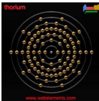
Rys 1. Schemat powłkowej struktury toru (nie jest to struktura atomu toru)[3].
