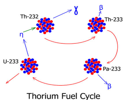
Rys 9. Schemat torowego cyklu i formowanie w ciała paliwowe paliwowego [18].
